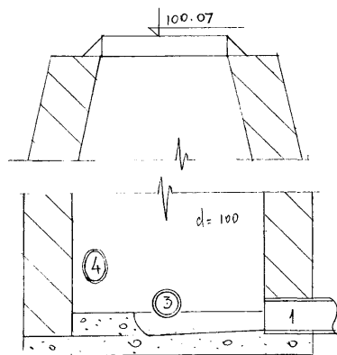
Чертеж колодца М 1:25
