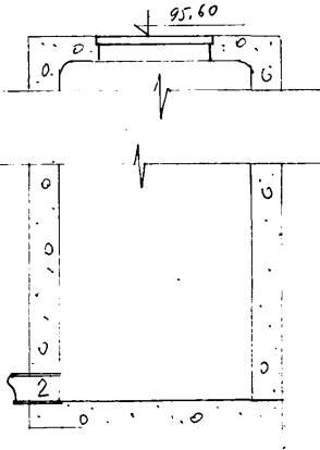
Чертеж колодца М 1:25
