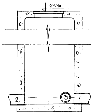
Чертеж колодца М 1:25
