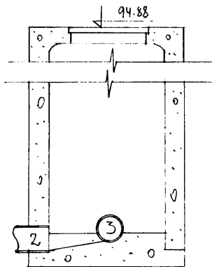
Чертеж колодца М 1:25
