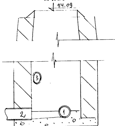
Чертеж колодца М 1:25
