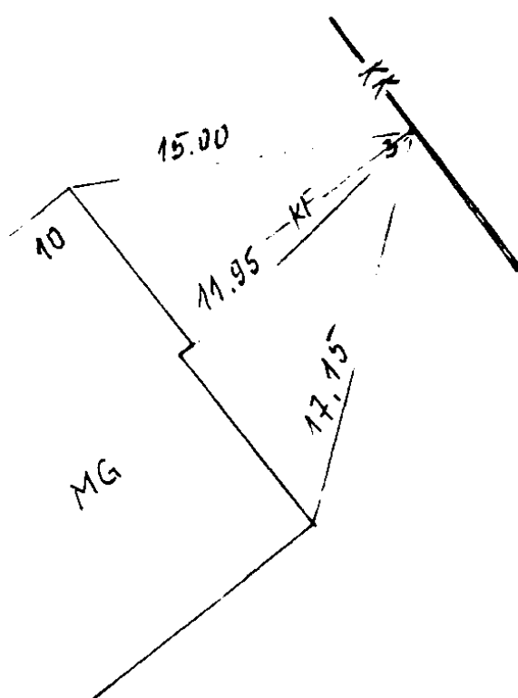
PRIRIŠIMO SCHEMA
