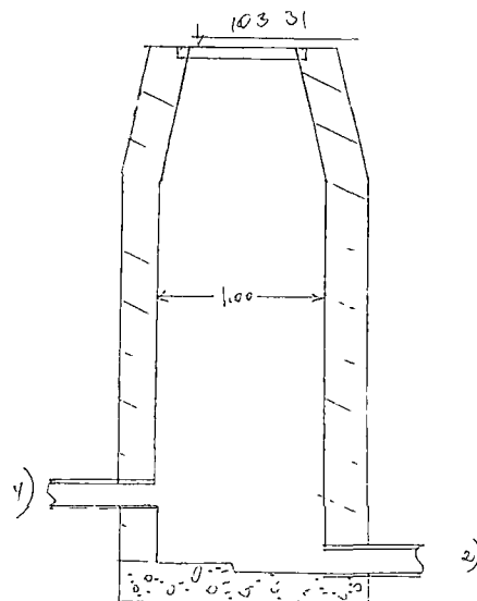
Чертеж колодца М 1:50
