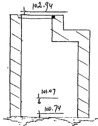
Чертеж колодца М. 1:50
