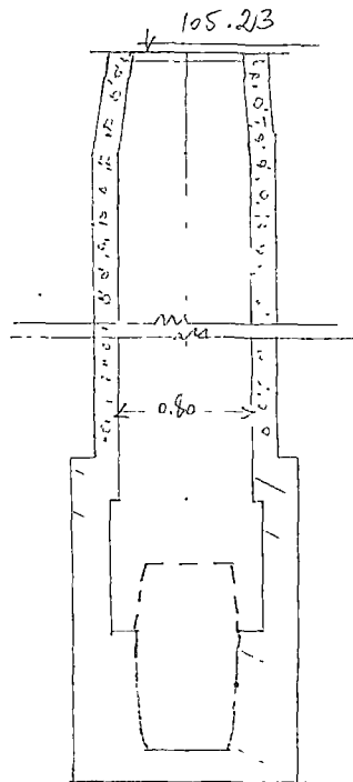
Чертеж колодца М 1:50
