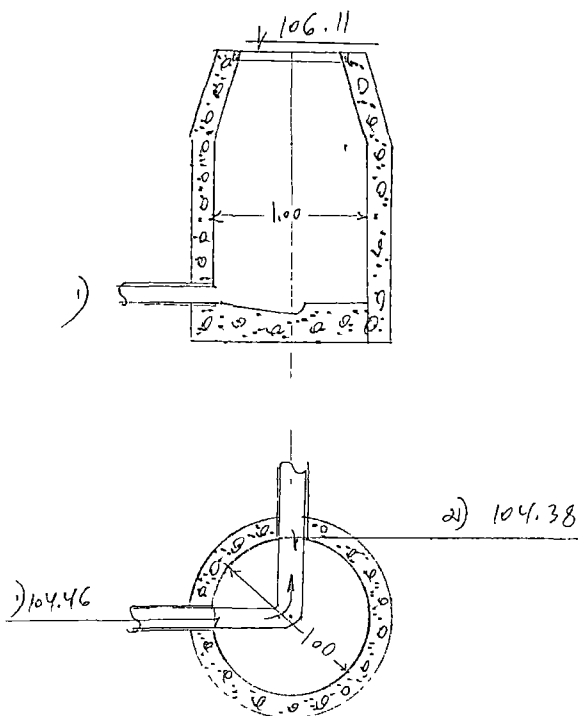
Чертеж колодца М 1:50
