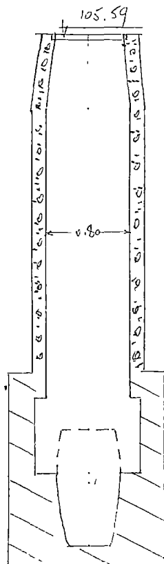
Чертеж колодца М 1:5
