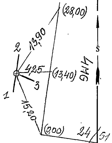
PRIRIŠIMO BRĖŽINYS
