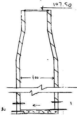
Чертеж колодца М 1:50
