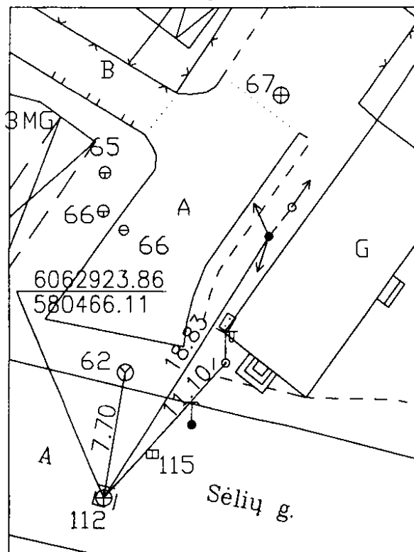
PRIRIŠIMO BRĖŽINYS
