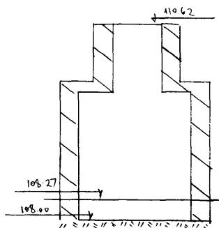
Чертеж колодца М. 1:50
