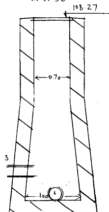
Чертеж колодца М 1:50
