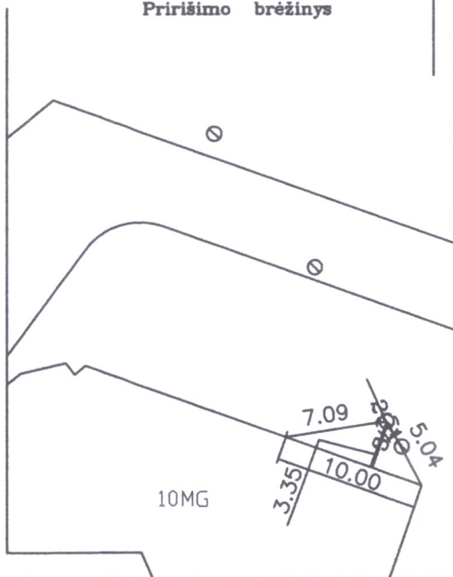
Pririšimo brėžinys
