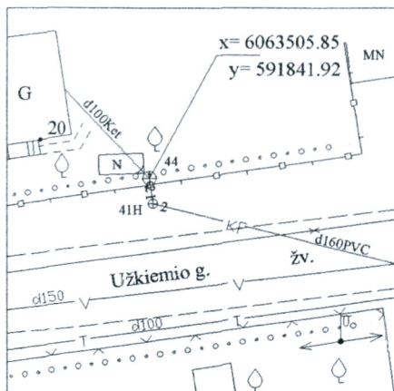
Pririšimo brėžinys
