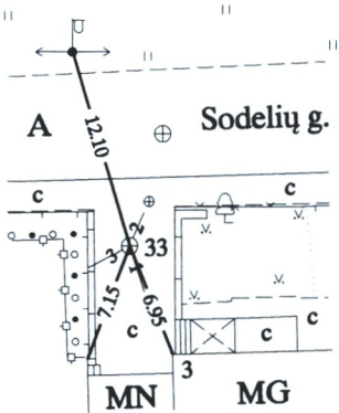
Pririšimo brėžinys :
