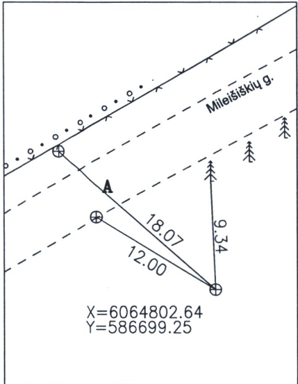
PRIRIŠIMO BRĖŽINYS
