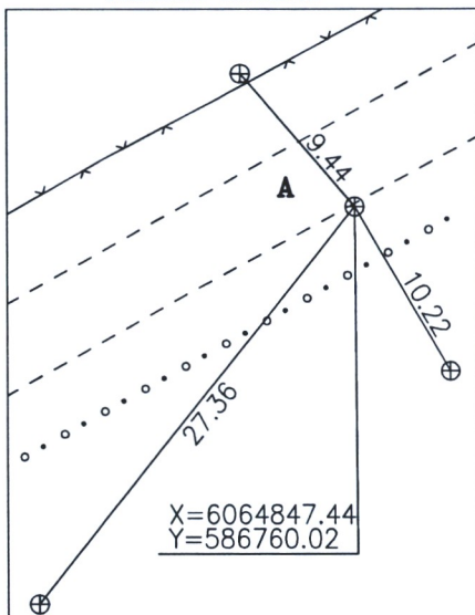
PRIRIŠIMO BRĖŽINYS
