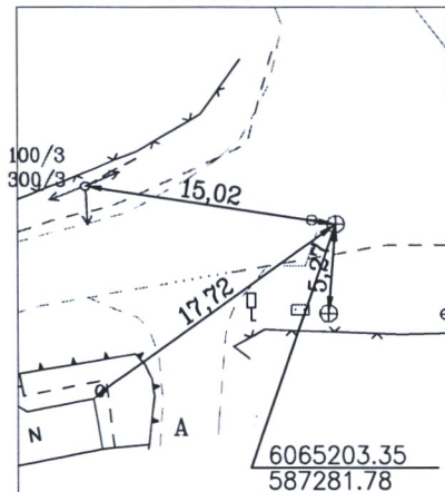
PRIRIŠIMO BRĖŽINYS
