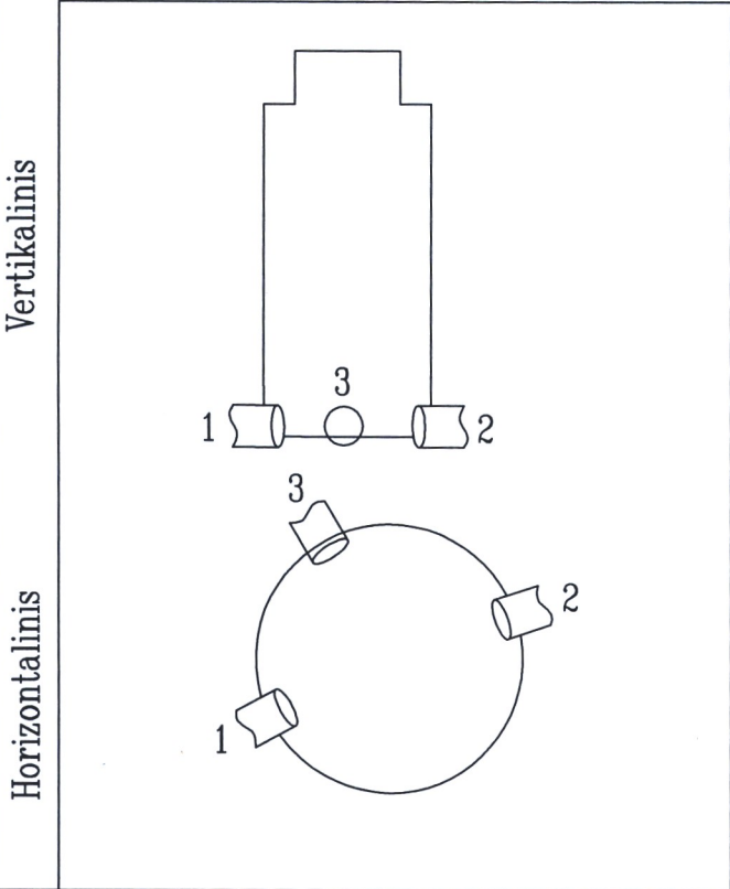
ŠULINIO PJŪVIAI (Matmenys duoti m)
