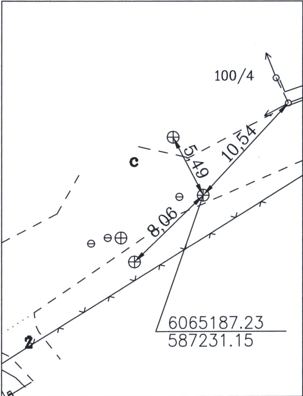
PRIRIŠIMO BRĖŽINYS
