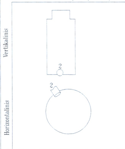
ŠULINIO PJŪVIAI (Matmenys duoti m)
