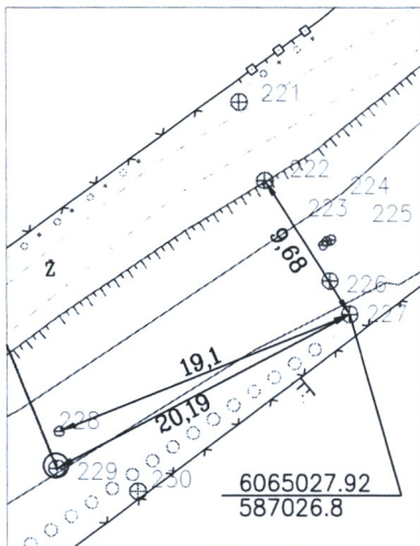
PRIRIŠIMO BRĖŽINYS
