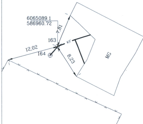
Pririšimo brėžinys :
