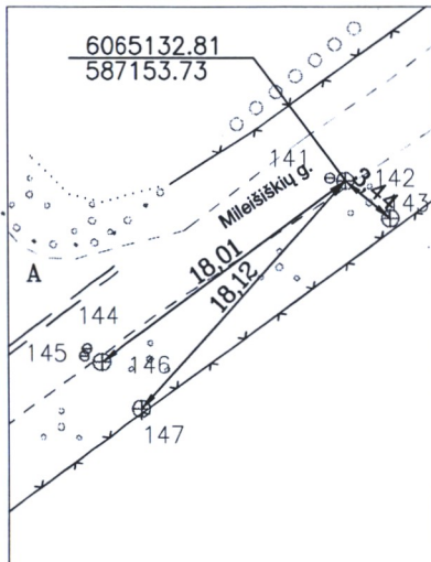
PRIRIŠIMO BRĖŽINYS
