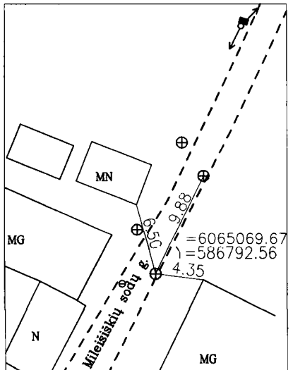
PRIRIŠIMO BRĖŽINYS
