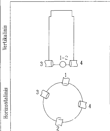
ŠULINIO PJUVIAI (Matmenys duoti m)
