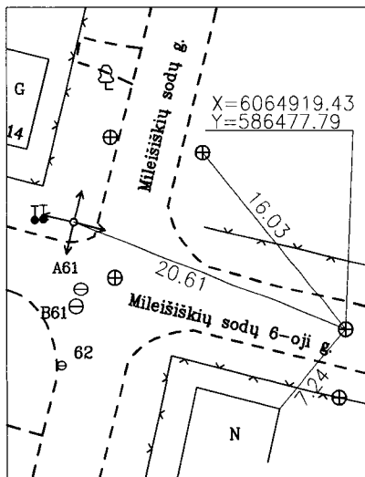
PRIRIŠIMO BRĖŽINYS
