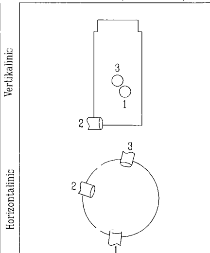
ŠULINIO PĖJIVIAI (Matmenys duoti m)
