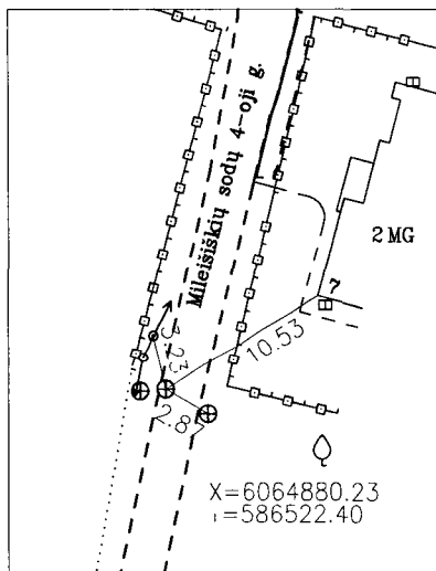
PRIRIŠIMO BRĖŽINYS
