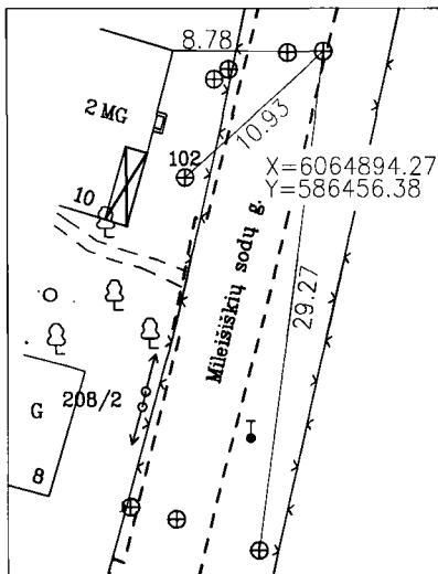
PRIRIŠIMO BRĖŽINYS
