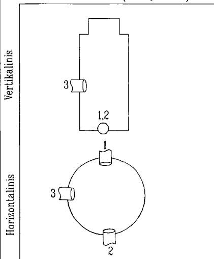
ŠULINIO PJOVIAI (Matmenys duoti m)
