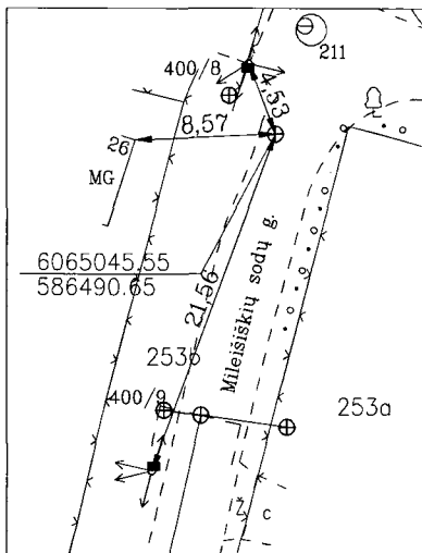
PRIRIŠIMO BRĖZINYS
