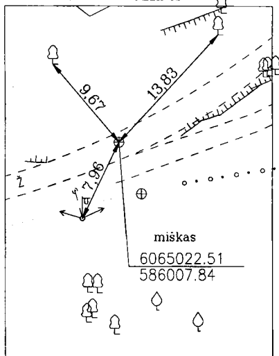
PRIRIŠIMO BRĖŽINYS
