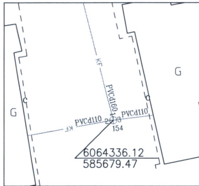
PRIRIŠIMO SCHEMA
