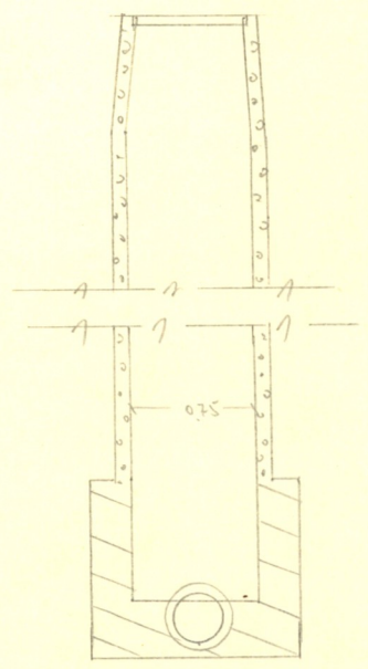
Чертеж колодца М 1:50 по А-А
