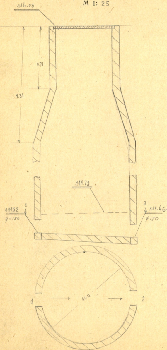
Чертеж колодца М 1:25
