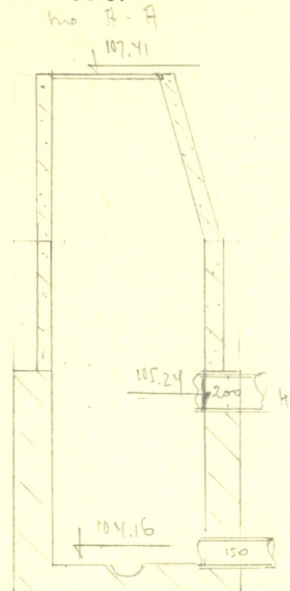
Чертеж колодца М 1:50
