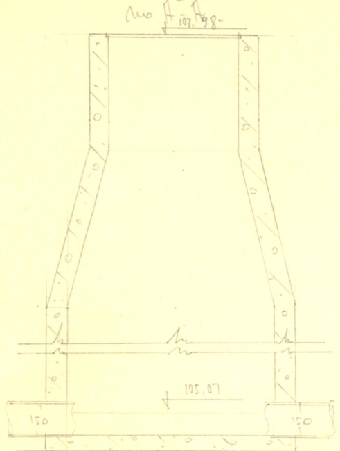
Чертеж колодца М 1:25
