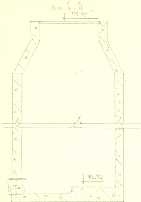
Чертеж колодца М 1:25
