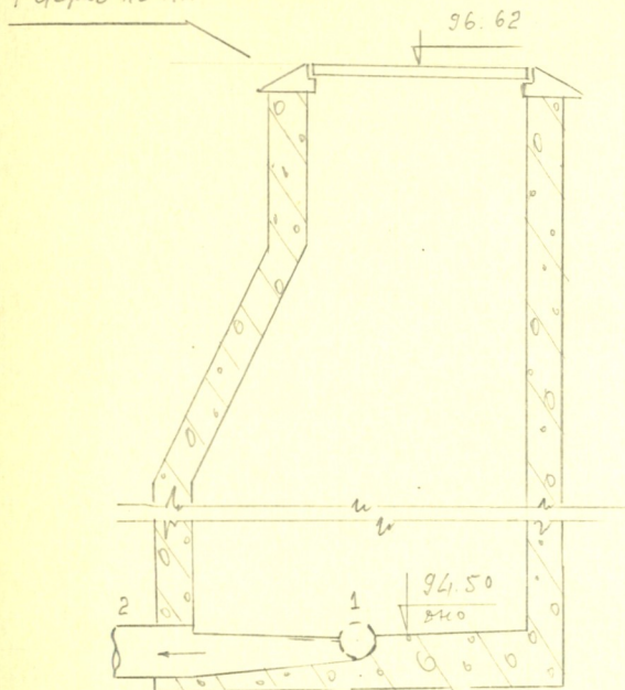
Чертеж колодца М 1:25 Разрез по АА
