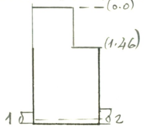
ŠULINIO PIŪVIAI (Matmenys duot. m)
