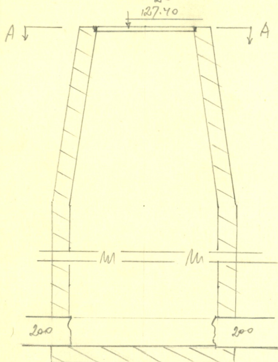
Чертеж колодца М 1:25
