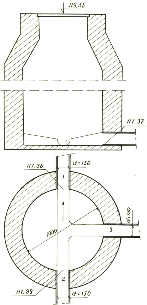
Чертеж колодца М 1:25
