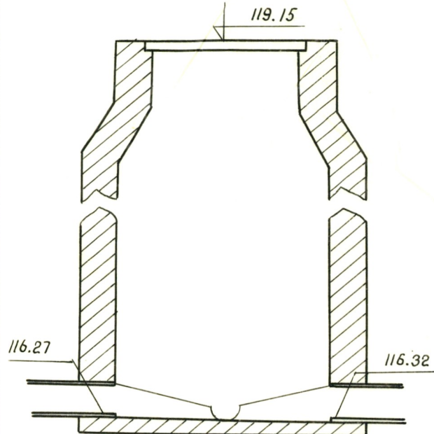
Чертеж колодца М 1:25
