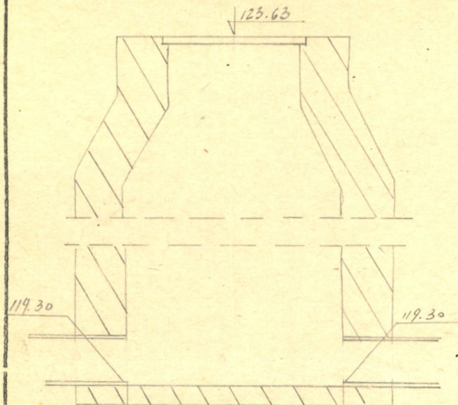
Чертеж колодца М 1:
