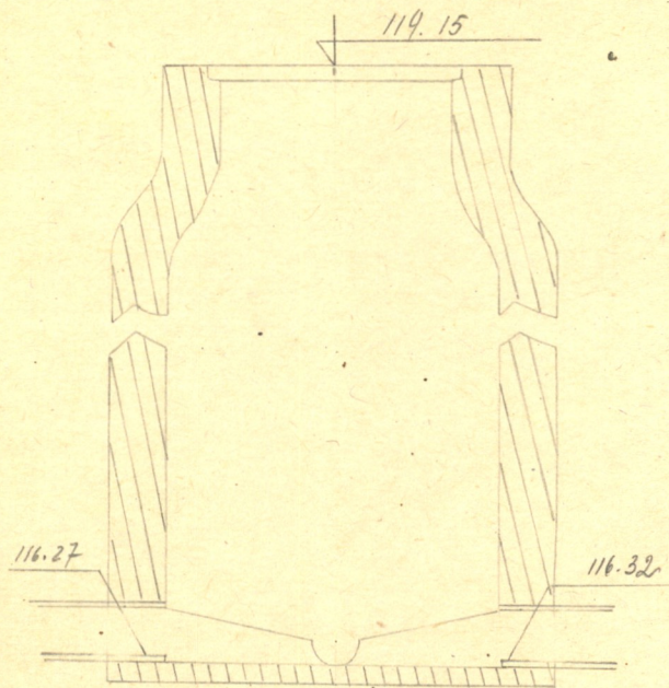
Чертеж колодца М 1:25
