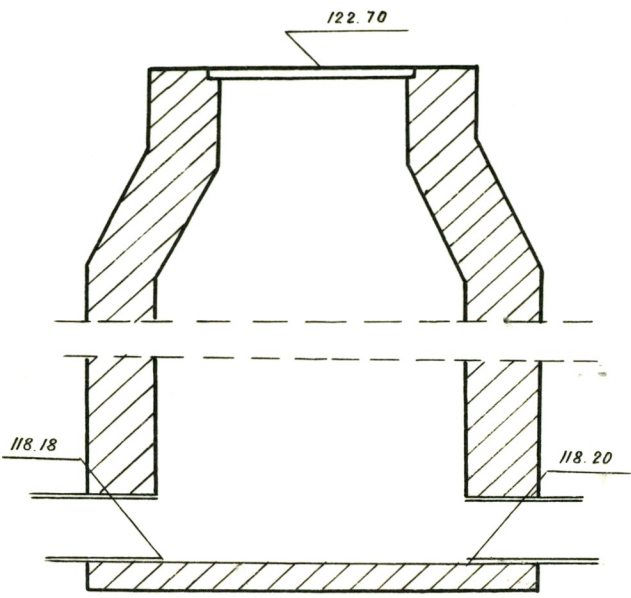
Чертеж колодца
