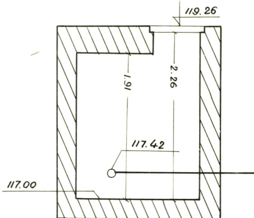
Чертеж колодца М 1:50
